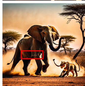
(j) +Attn-SF
